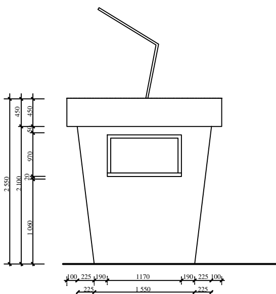
Вид спереди
