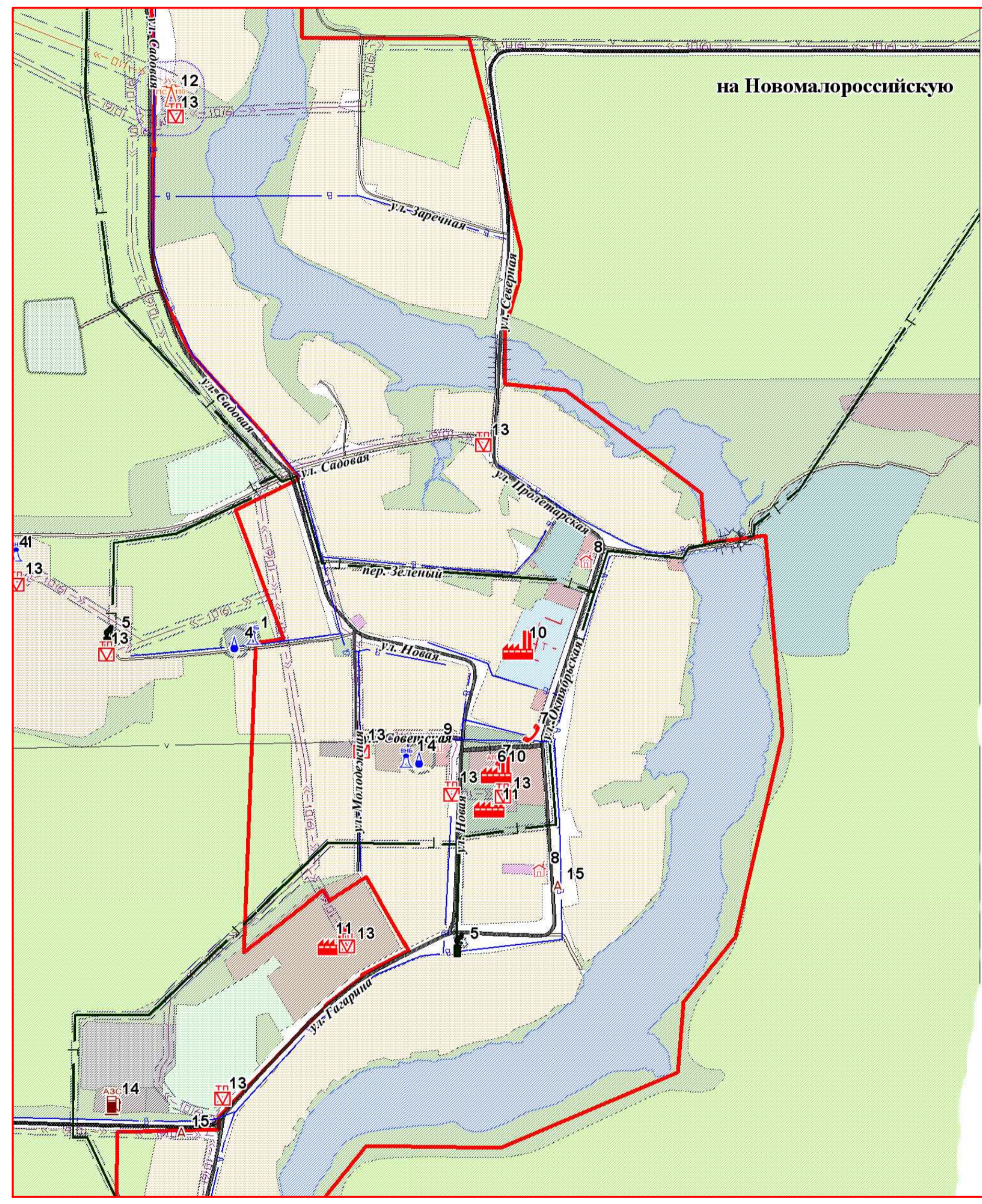
Схема теплоснабжения станции Бузиновская фрагмент территории
