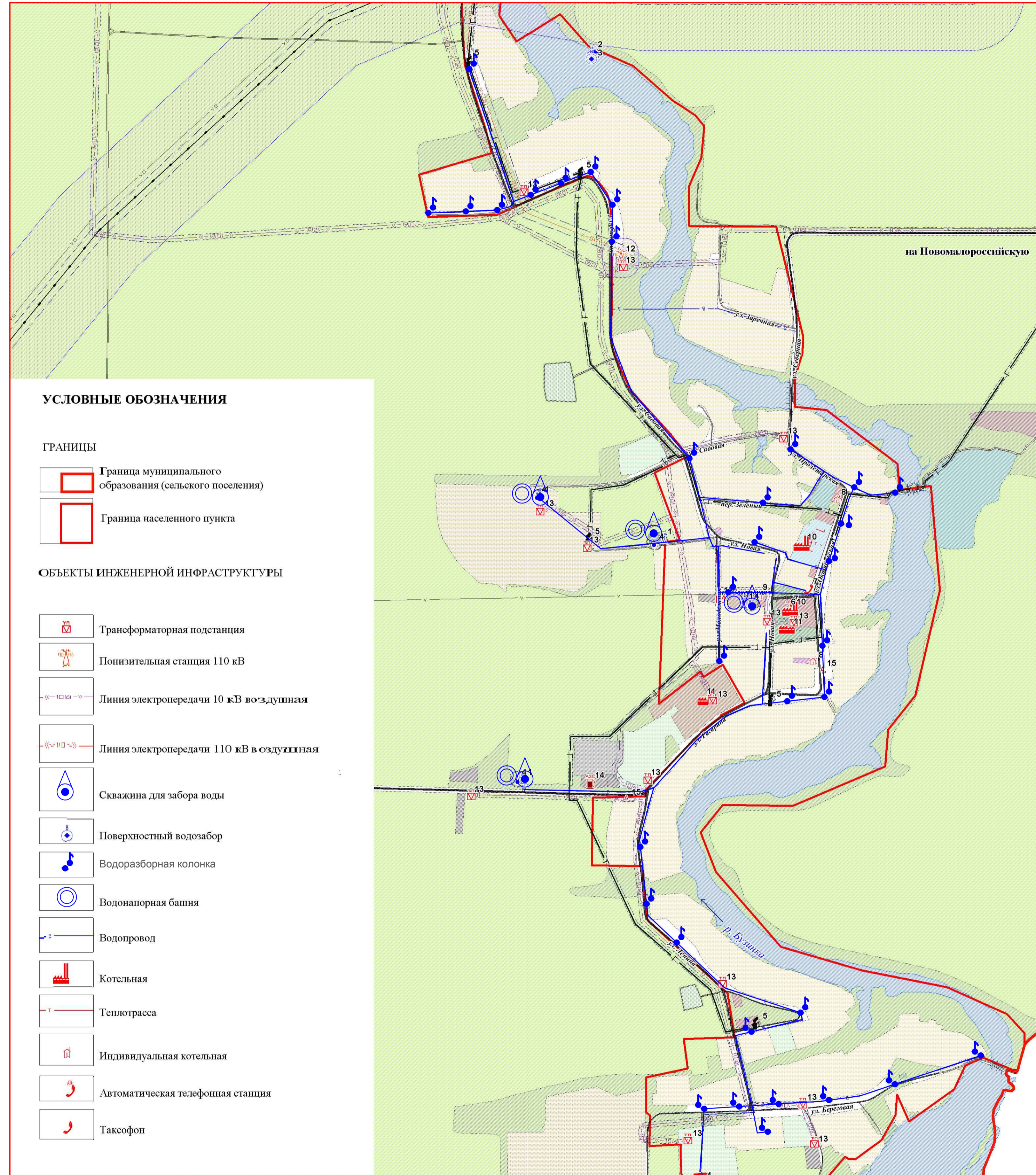
Схема водоснабжения станицы Бузиновская центральная и южная часть фрагмент территории
