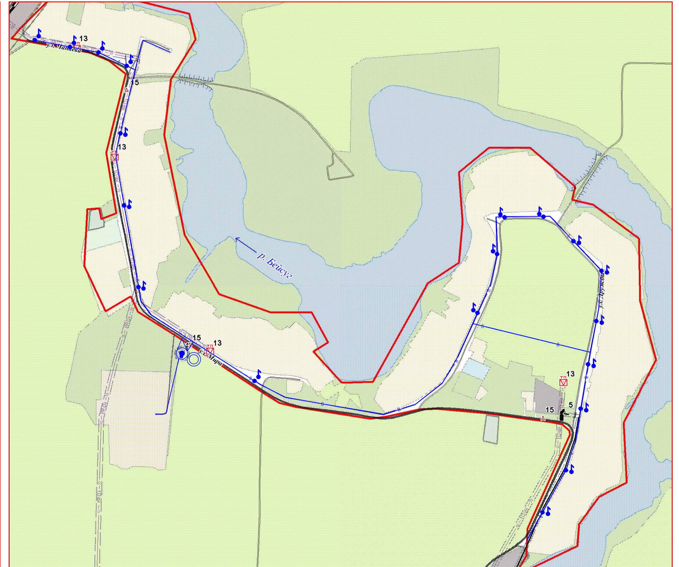
Схема водоснабжения станицы Бузиновская северная часть фрагмент территории
